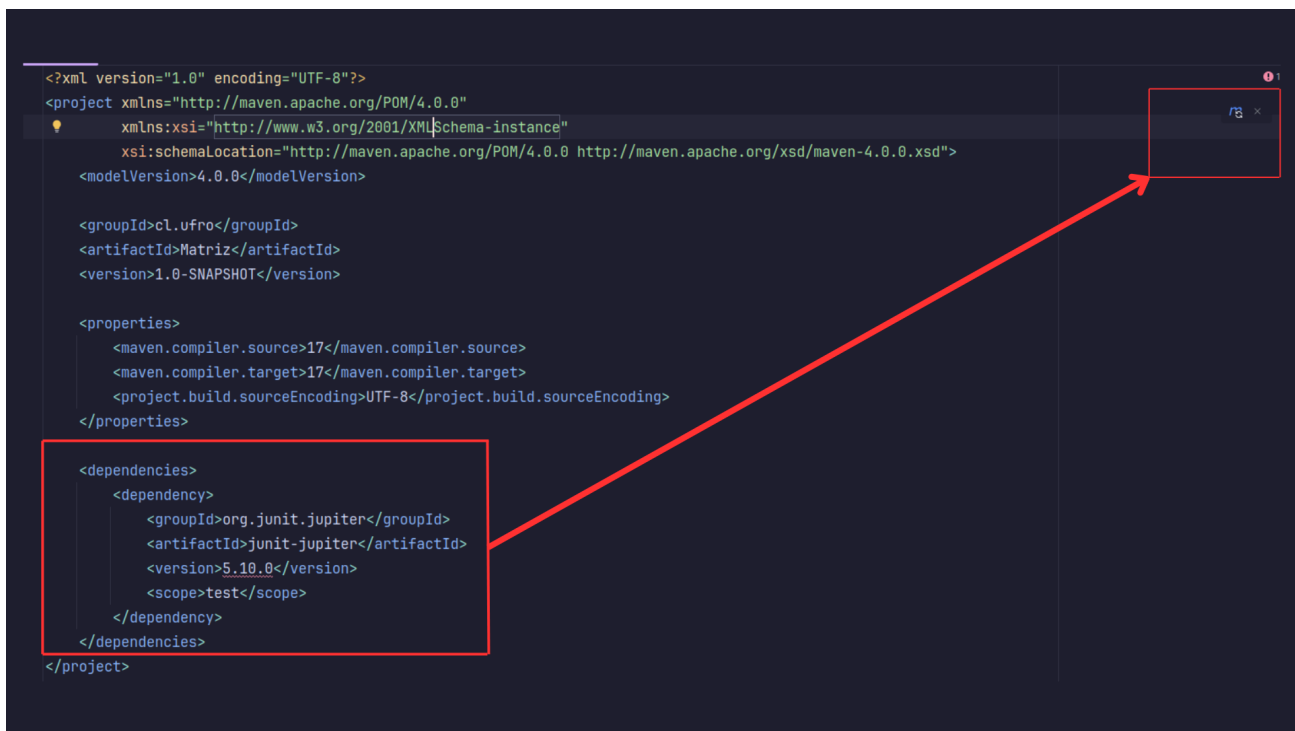
Figura 6: Sincronización del archivo pom.xml con Maven
